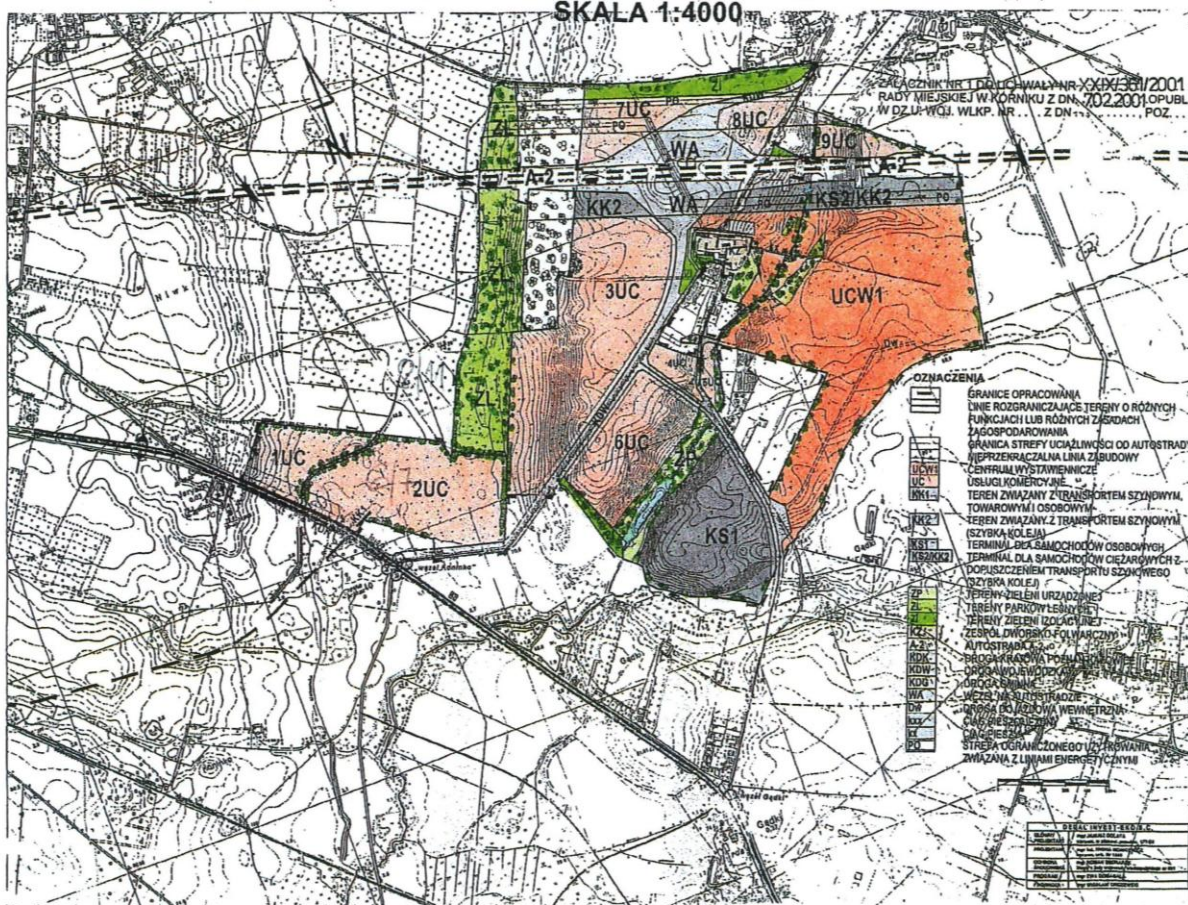
MIEJSCOWY PLAN ZAGOSPODAROWANIA PRZESTRZENNEGO OBSZARU USŁUG KOMERCYJNYCH W ŻERNIKACH, GMINA KÓRNIK SKALA 1:4000
