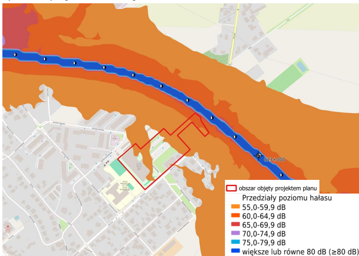
Ryc. 4. Tereny zagrożone hałasem wg wskaźnika LDWN 15
